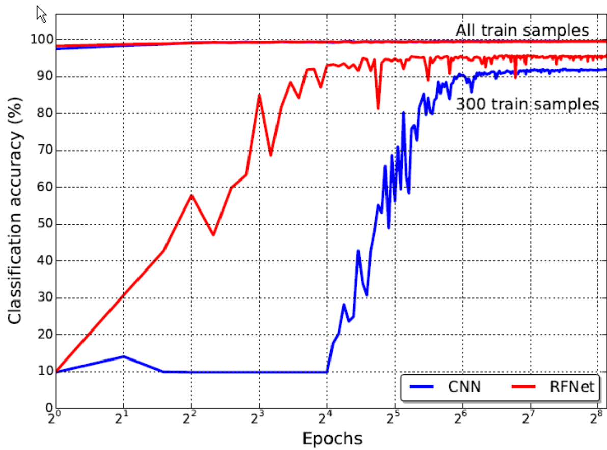
(b) MNIST
